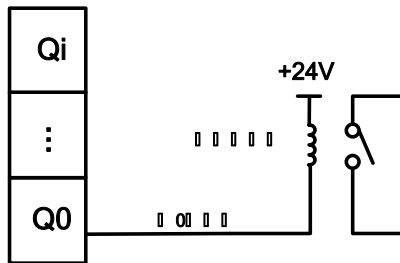
图 4-2-15 数字量输出接线方法
