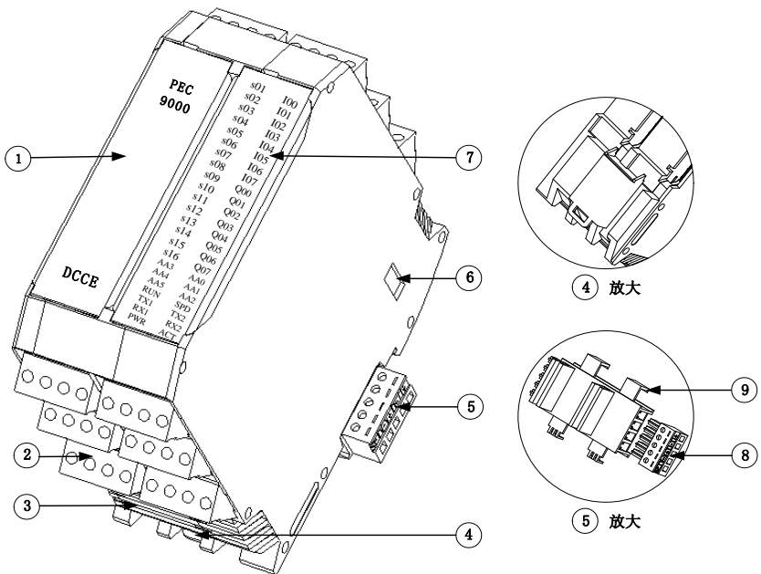
图 4-1-1 整体外观
