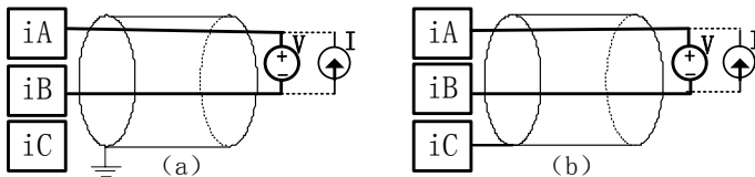
图 4-2-11 电压型有源输入接线方法
