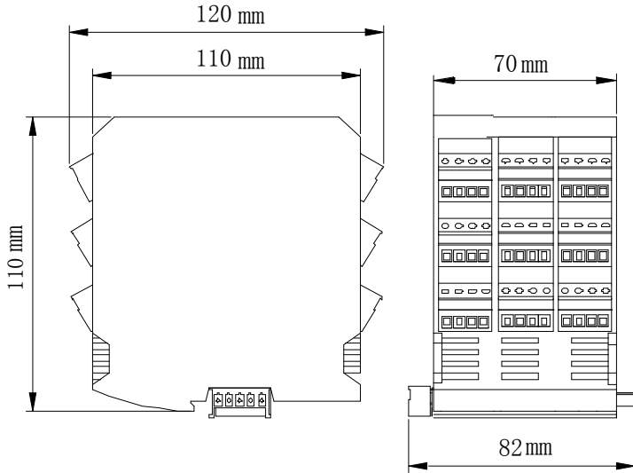
图 4-1-2 外形尺寸
