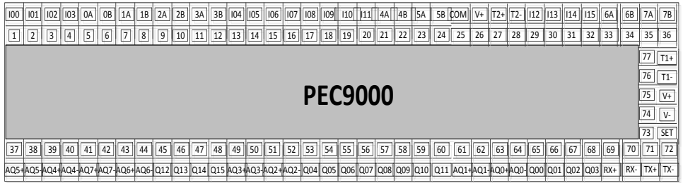
图 4-2-2 PEC9000 原理图
