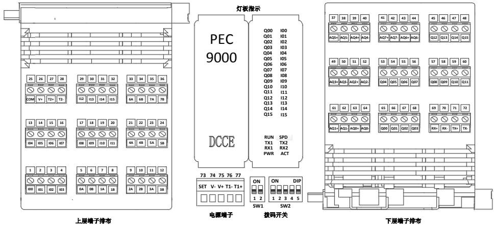
图 4-2-1 端子位置排布
