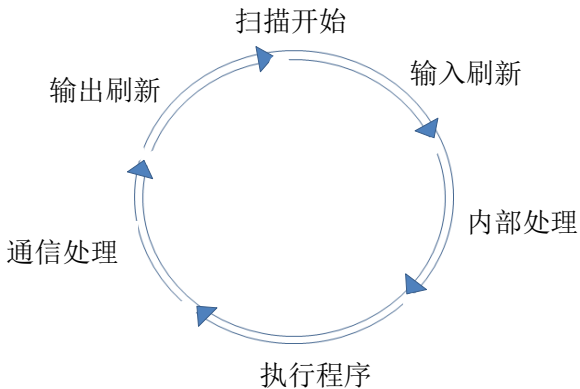
图5-2-7扫描周期
