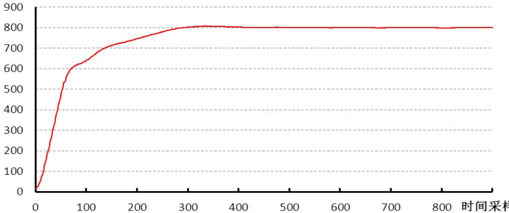
图 5-2-4 P_PID 无过冲自整定控温曲线图
