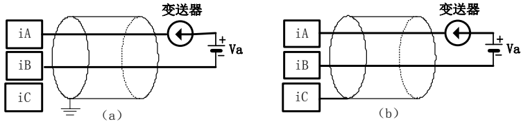
图 4-2-12 电流型无源输入接线方法
