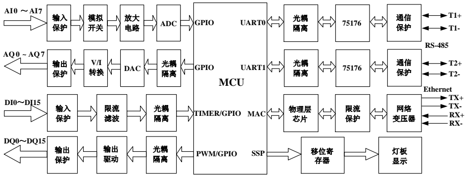
图 2-1-1 PEC9000 原理框图
