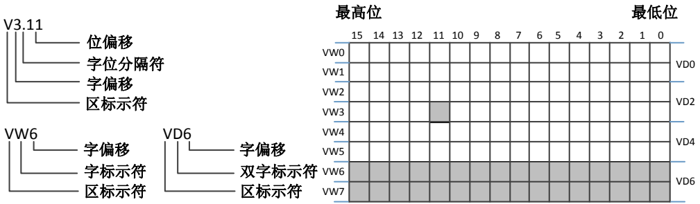
图5-2-1变量寻址示意图
