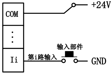
图 4-2-14 数字量输入接线方法
