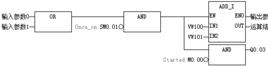
图 5-2-9 功能块编程语言
