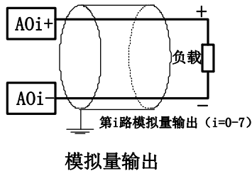
图 4-2-13 模拟量输出接线方法
