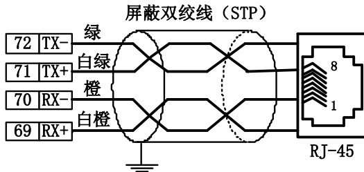
图 4-2-8 以太网接线方法
