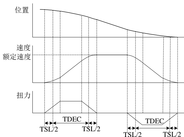
图 6-2-4 位置 S 曲线与时间设定关系（位置指令减少）
