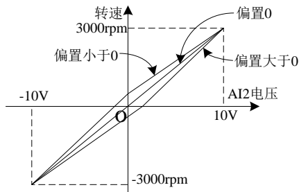
图 7-7-3 AI2 采样偏置图
