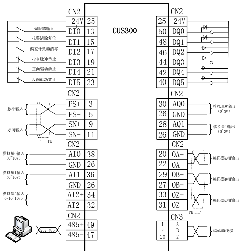
图 4-2-1 位置模式接线图
