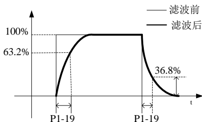
图 6-3-3 低通滤波曲线
