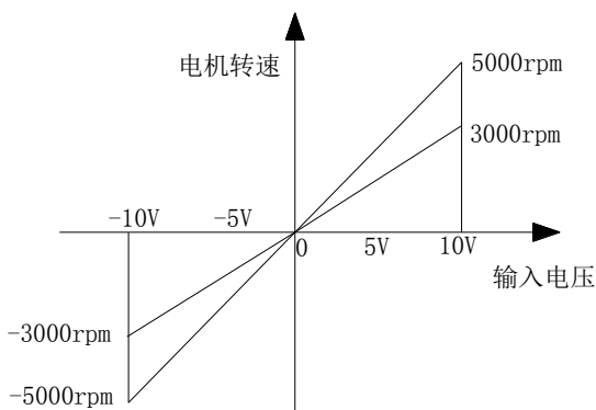
图 6-3-4 指令增益特性
