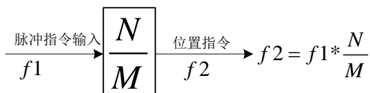
图 6-2-1 位置控制基本框图
