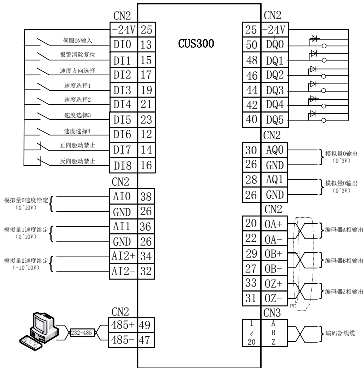
图 4-2-2 速度模式接线图
