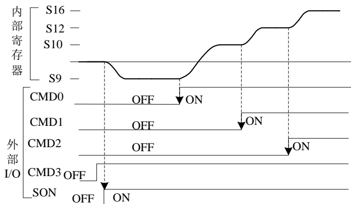
图 6-3-5 外部 DI 与速度内部指令寄存器关系
