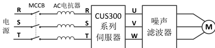
图 4-4-2 主回路电机侧连接图
