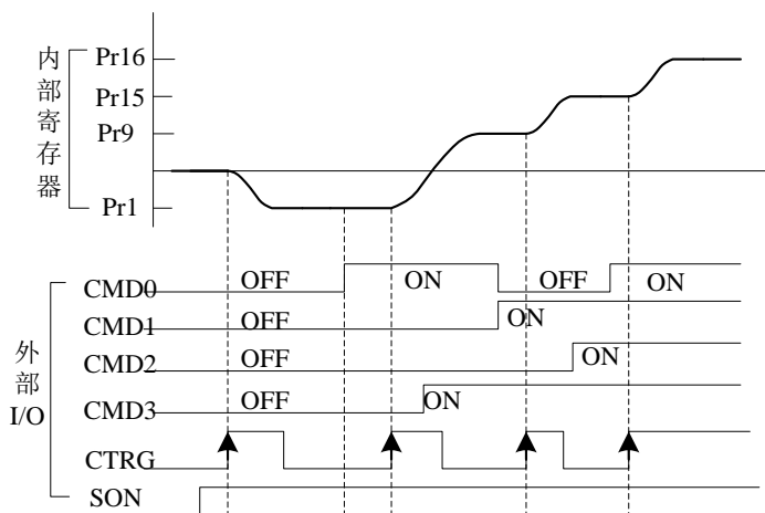
图 6-2-5 外部 DI 与 P2 在寄存器的关系
