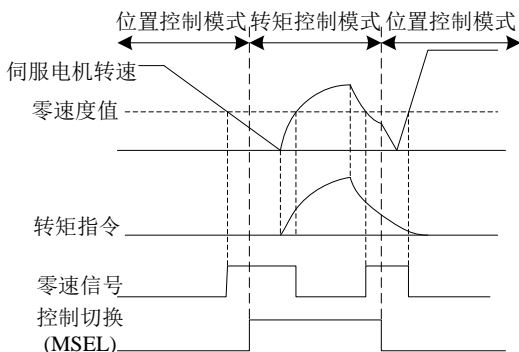
图 6-5-3 速度位置切换图示
