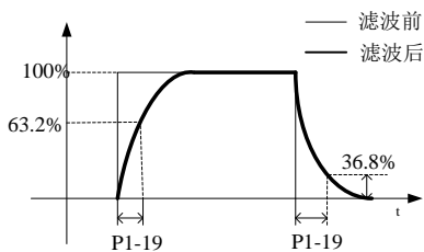
图 7-2-3 低通平滑滤波图
