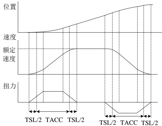
图 7-2-1 位置 S 曲线图 (指令增加)
