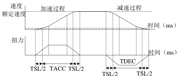
图 6-3-2 速度指令与时间参数设定关系
