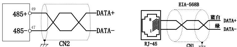
图 4-5-1 RS-485 接线方式
