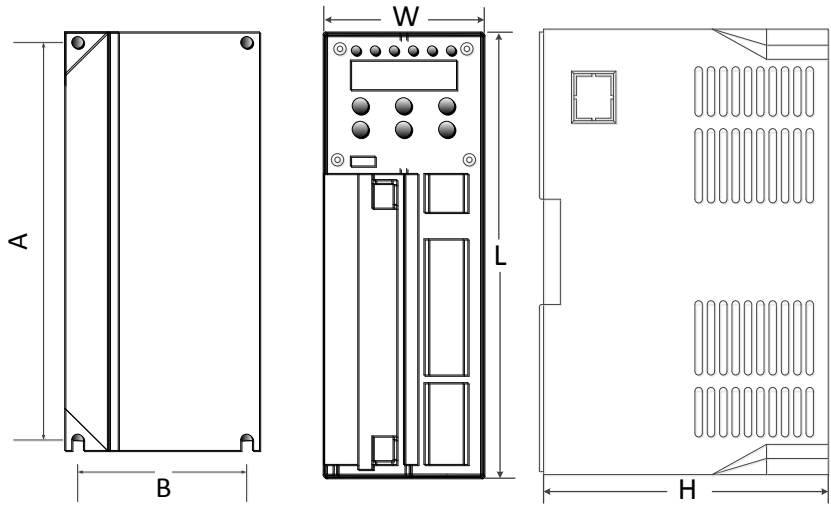
图 1-5-1 机型及打孔尺寸
