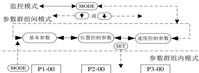
图 5-2-3 参数群组操作
