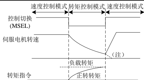
图 6-5-2 速度转矩切换图示
