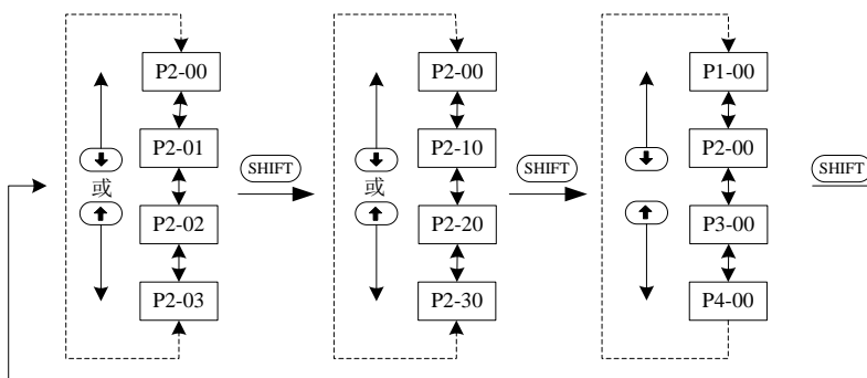
图 5-2-4 参数群组内操作
