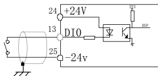
图 4-5-2 数字量输入接线
