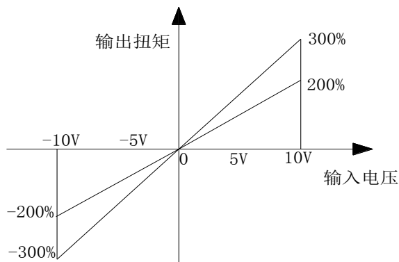
图 6-4-3 指令增益特性
