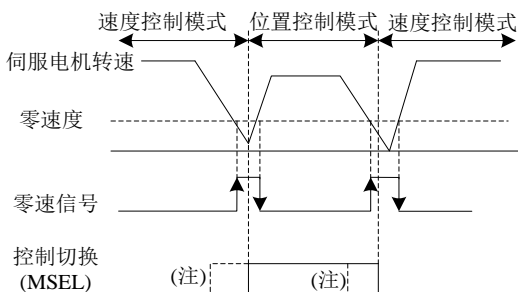
图 6-5-1 速度位置切换图示
