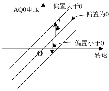
图 7-7-4 AQ0 输出偏置调整图
