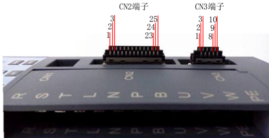
图 4-1-2 前视图端子序号定义
