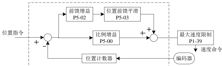
图 6-2-6 位置指令控制单元
