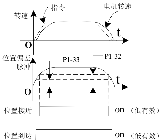
图 7-2-5 定位接近/完成信号图
