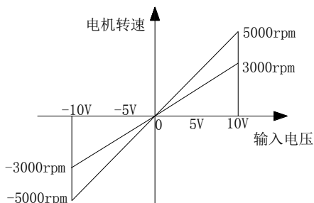
图 7-2-4 模拟速度指令增益图
