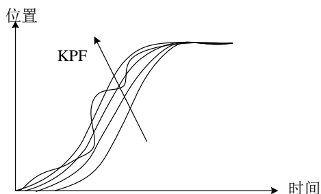
图 6-2-7 b 位置前馈增益
