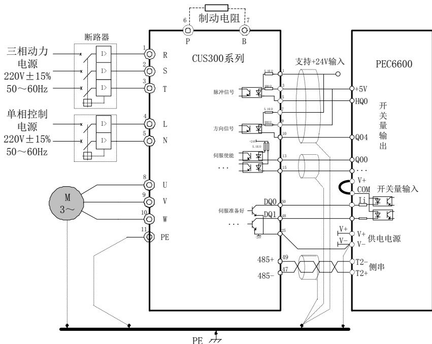
图 4-2-4 与 PLC 连接典型接线图
