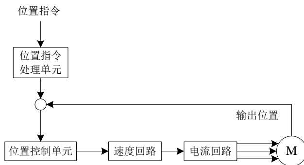
图 6-2-1 位置控制基本框图
