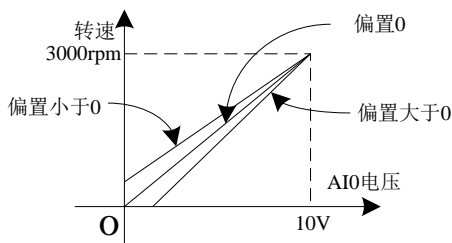
图 7-7-1 AI0 采样偏置图
