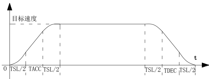
图 7-2-2 速度 S 曲线图
