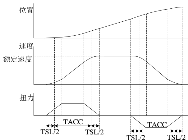
图 6-2-3 位置 S 曲线与时间设定关系（位置指令增加）
