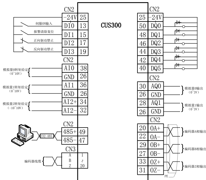
图 4-2-3 转矩模式接线图
