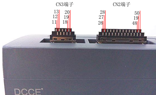
图 4-1-3 后视图端子序号定义
