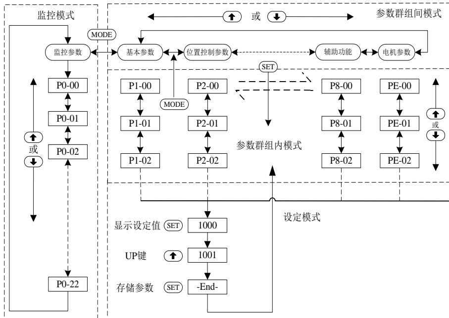
图 5-2-1 参数设置流程图
