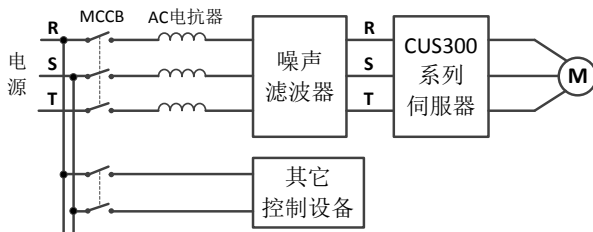
图 4-4-1 输入侧噪声滤波器接线方式
