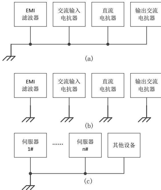
图 4-6-1 伺服驱动器附件接地方法
