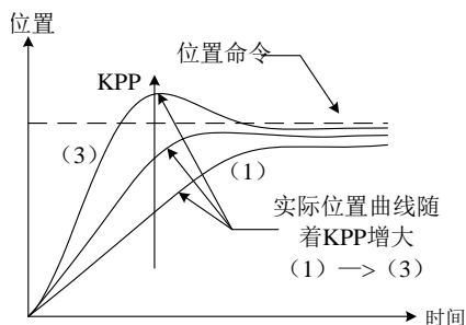
图 6-2-7 a 位置比例增益
