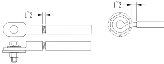
图 4-3-1 多芯线和单芯线压线方式
