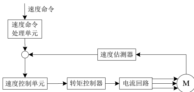
图 6-3-1 速度控制基本构架
