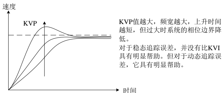
图 6-3-6.a 速度比例增益时域特性
