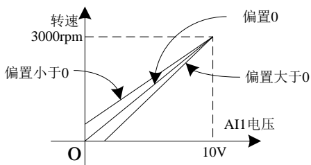
图 7-7-2 AI1 采样偏置图
