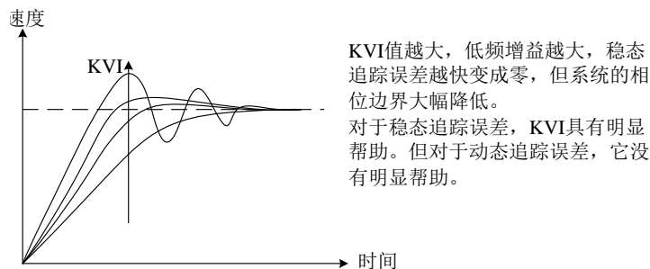
图 6-3-6.b 速度积分增益时域特性
