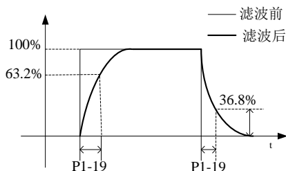
图 6-4-2 低通滤波曲线
