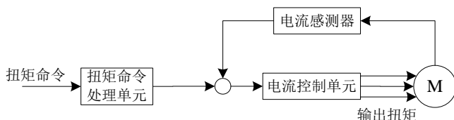
图 6-4-1 转矩模式基本结构
