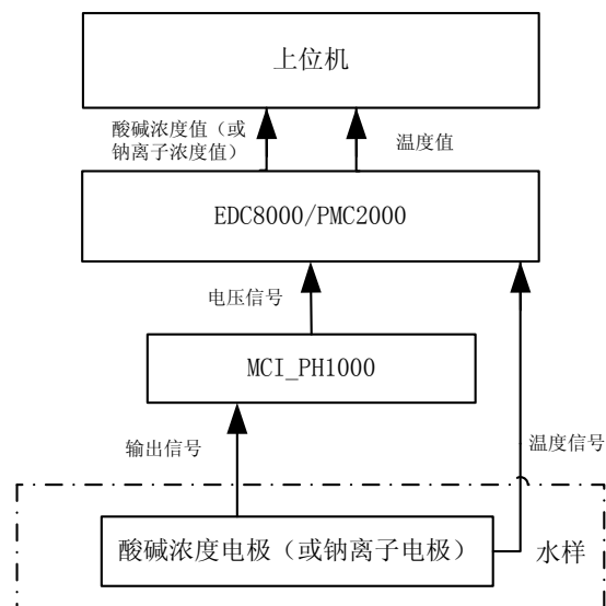
图 2-1 系统结构框图
