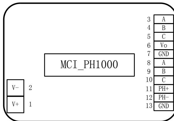
图 4-2-1 MCI_PH1000/MCI_NA1000 端子位置排布
