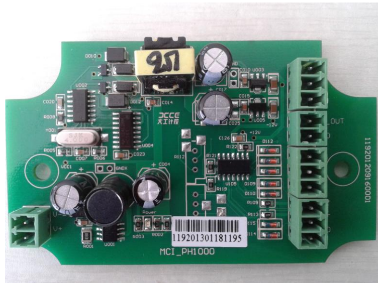
图 4-2-1 MCI_PH1000 实物图
