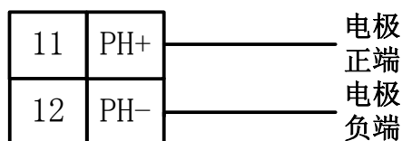
图 4-2-5 电极信号输入接线
