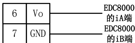
图 4-2-6 调理信号输出接线
