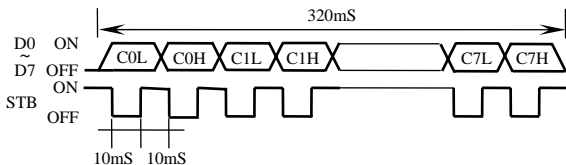
图 9 无条件字节输出上升沿选通时序
