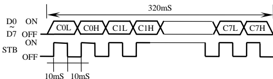
图 10 无条件字节输出下降沿选通时序
